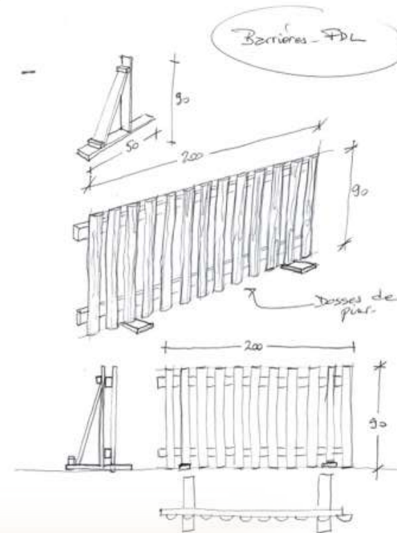
Barrières bois brut Quantité x 330ml Dimensions: hauteur 80cm x Largeur 200 cm
